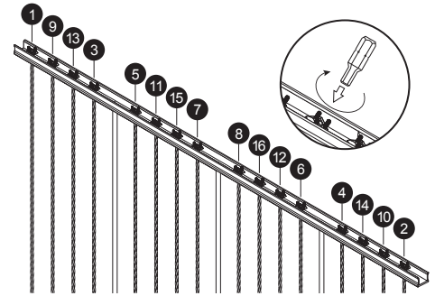
Dia. 8
