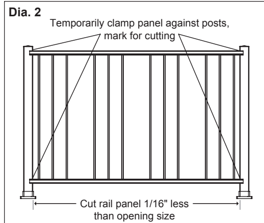
Dia. 2
