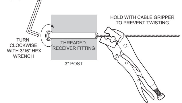
Dia. 8
