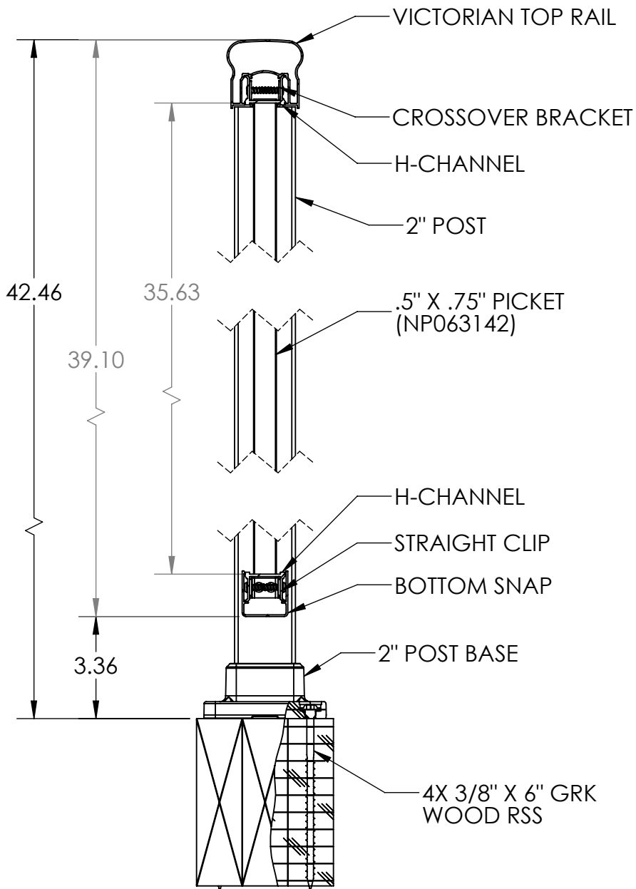
SECTION A-A
