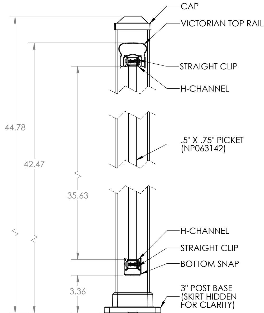
SECTION A-A
