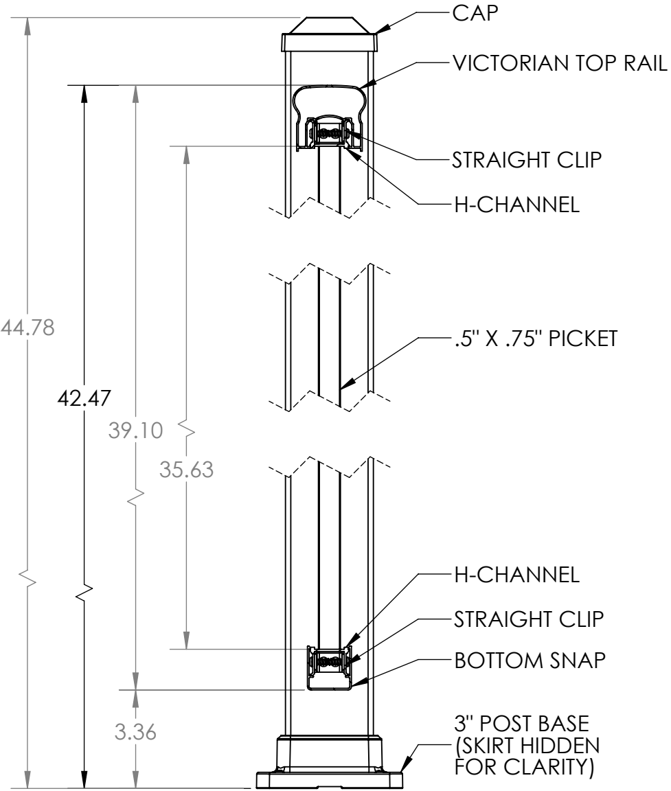
SECTION A-A
