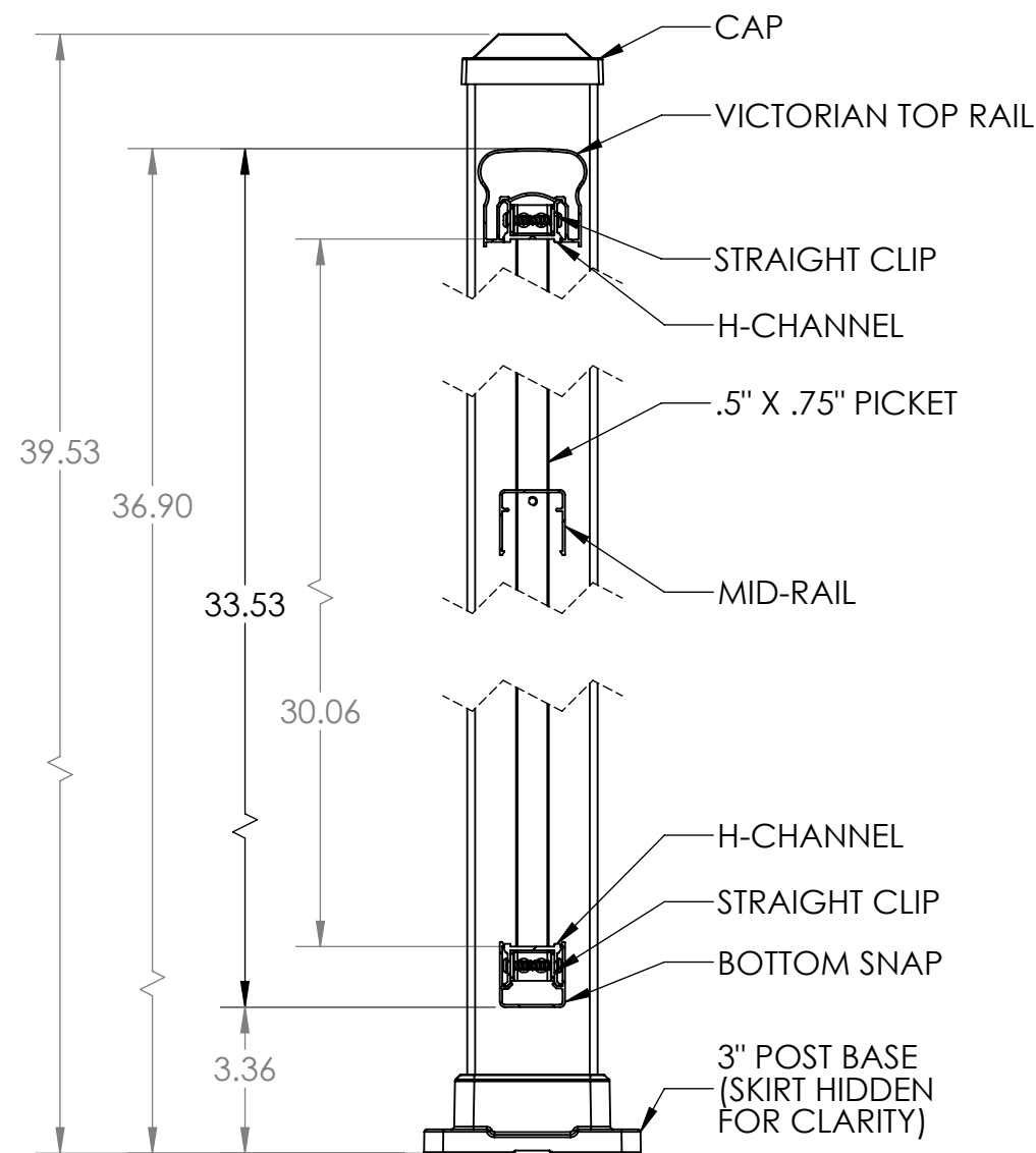
SECTION A-A
