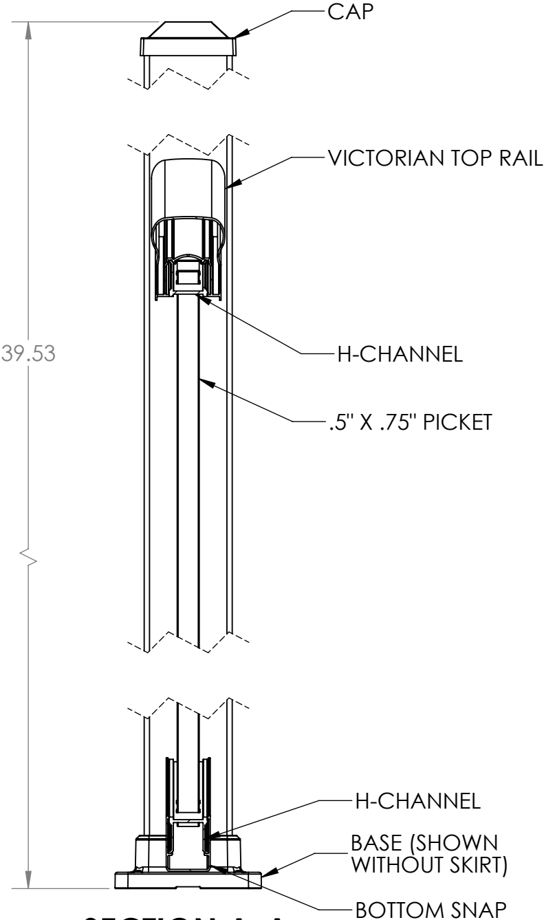
SECTION A-A
