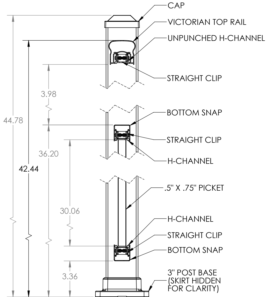
SECTION A-A
