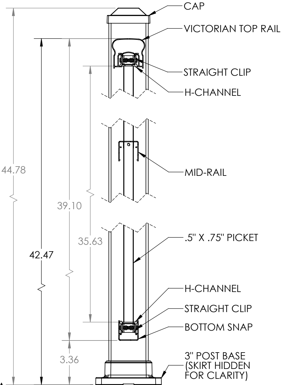
SECTION A-A
