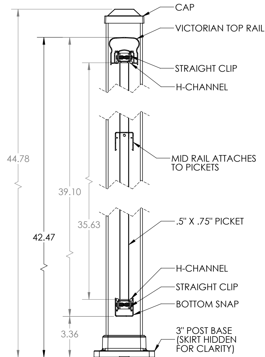
SECTION A-A
