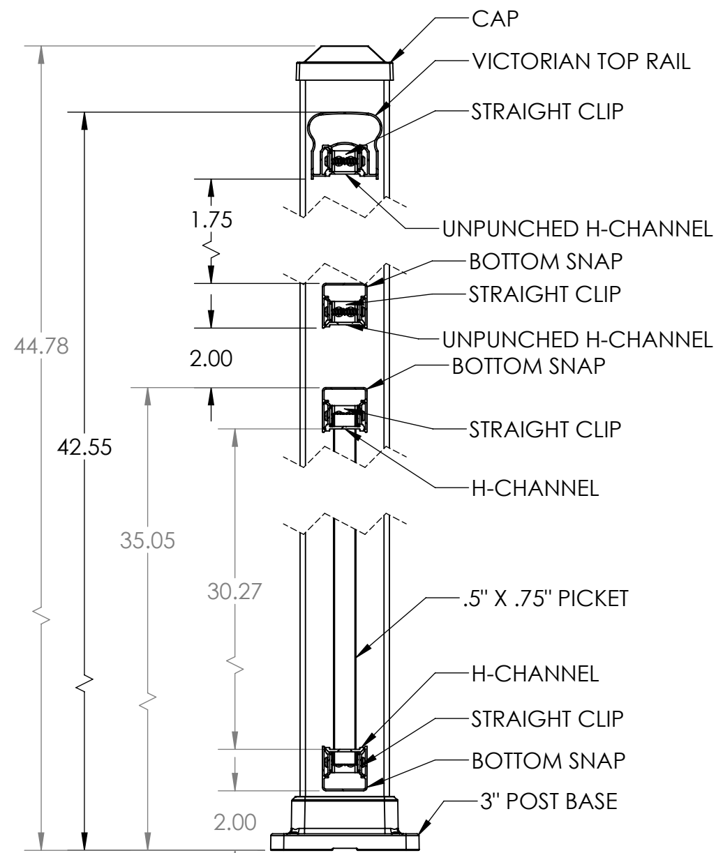
SECTION A-A
