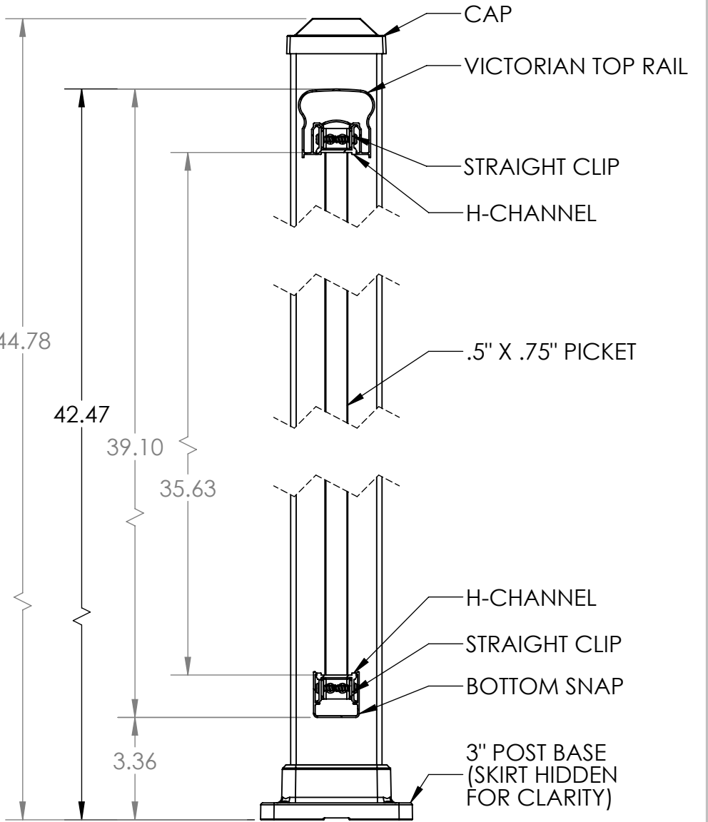
SECTION A-A
