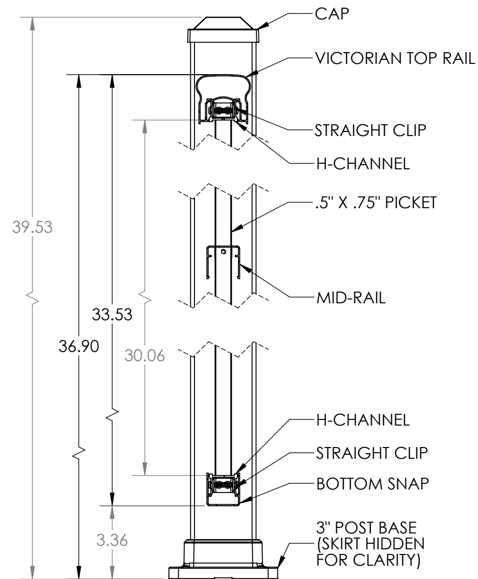
SECTION A-A
