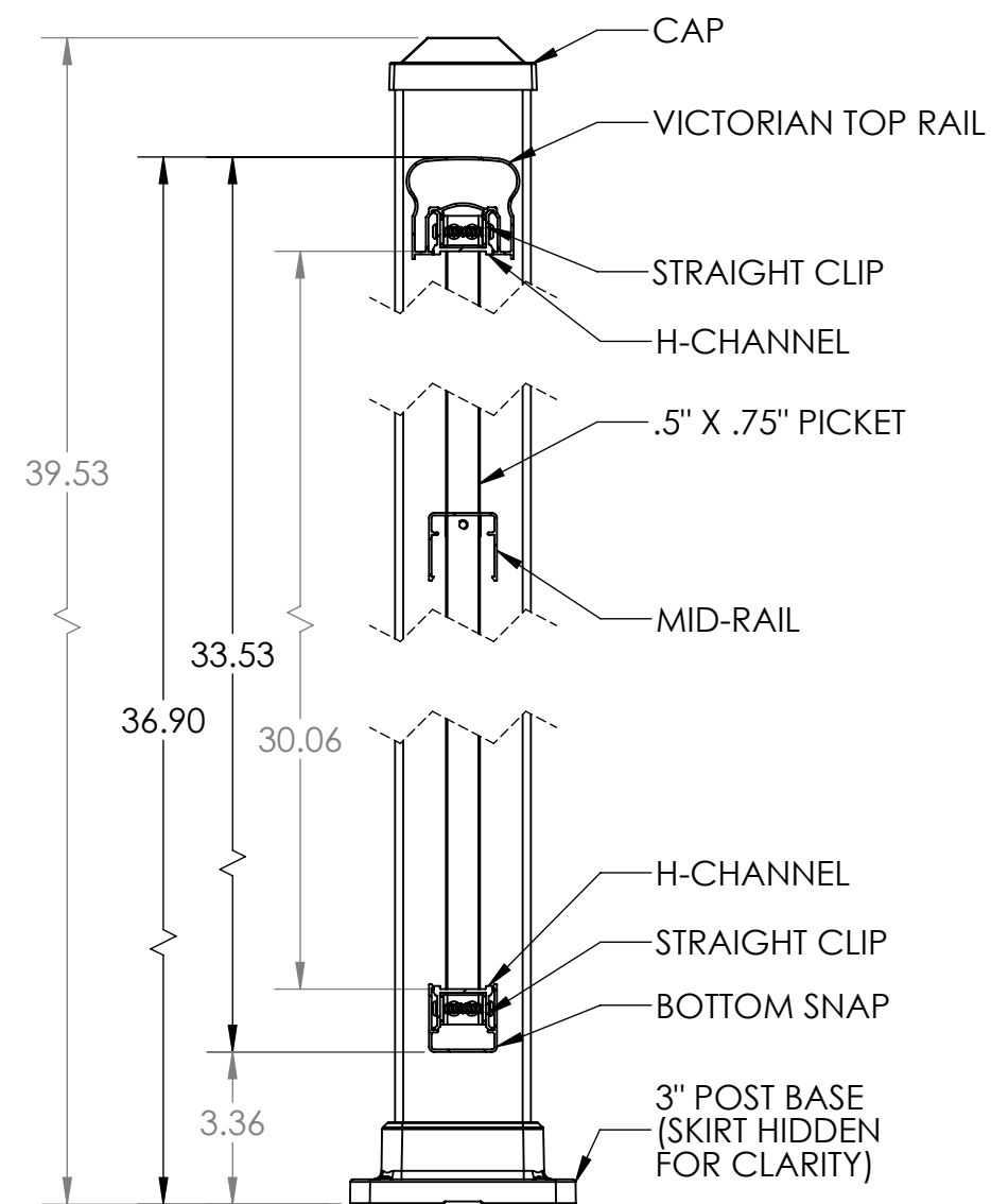
SECTION A-A
