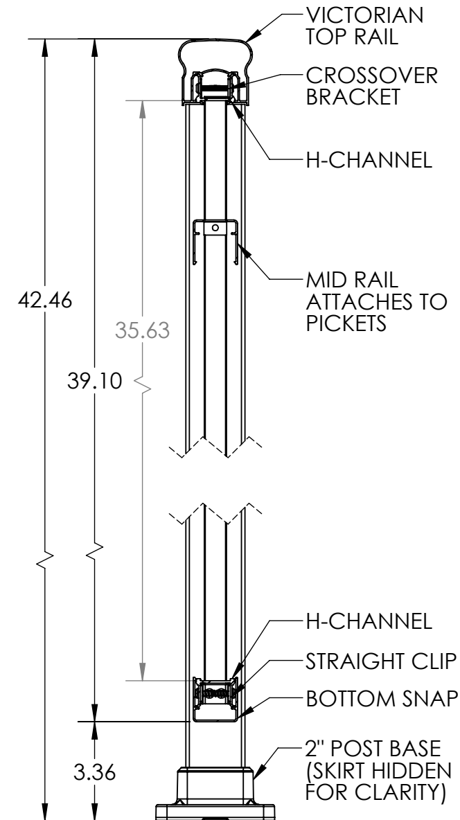
SECTION A-A
