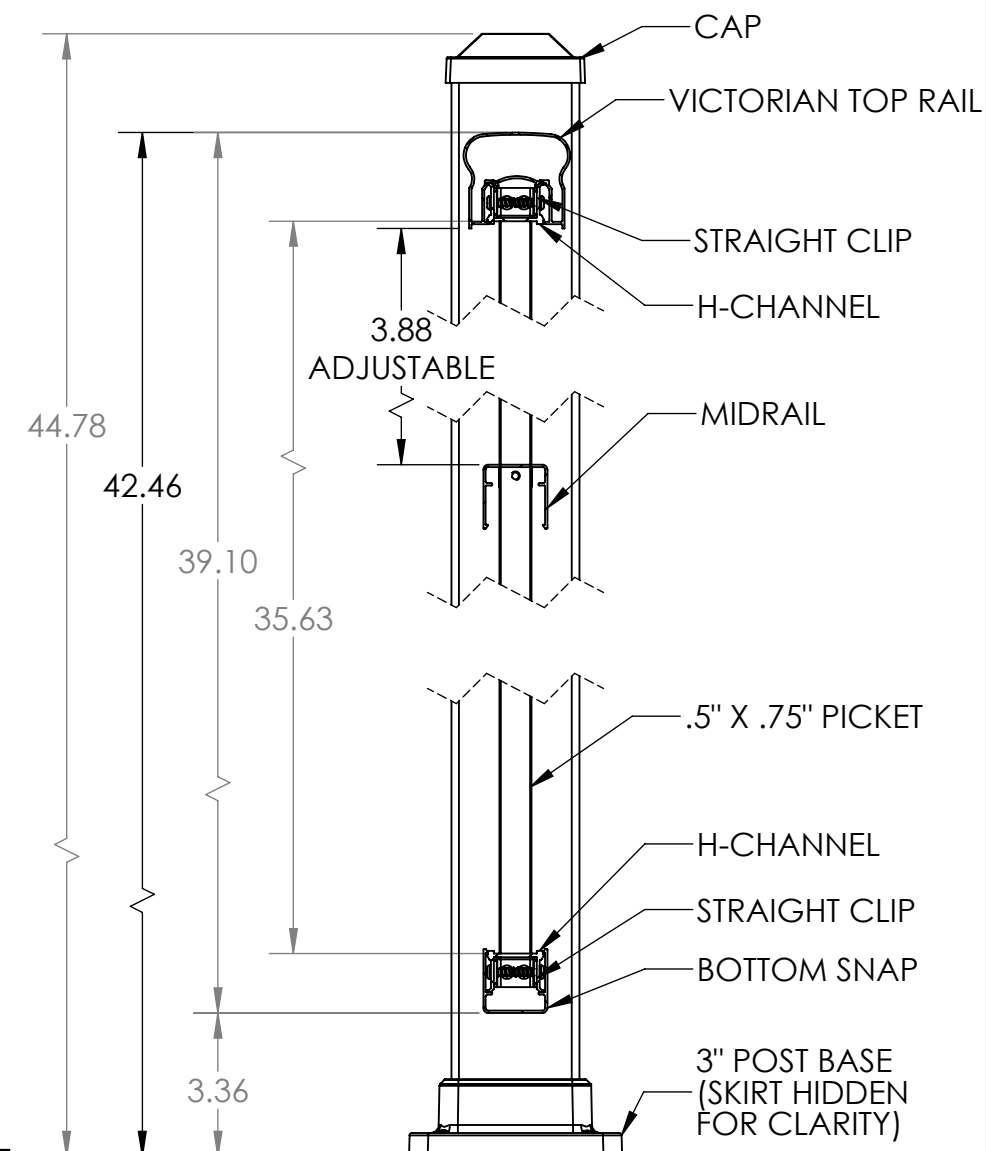
SECTION A-A
