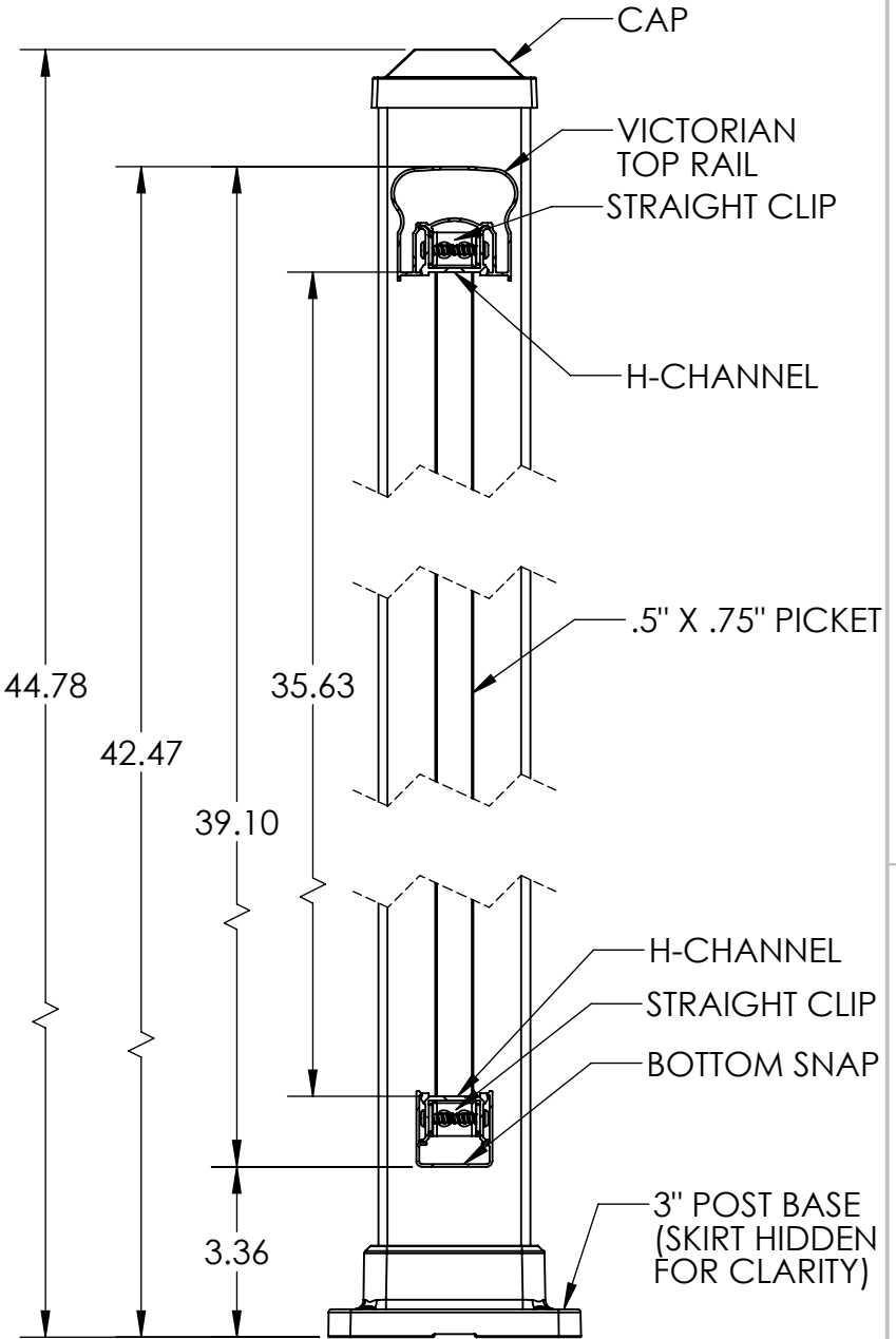
SECTION A-A
